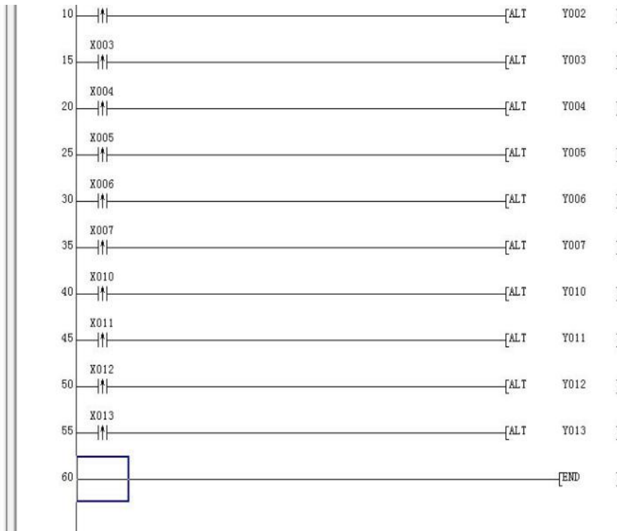
编写的几个简单PLC梯形程序
